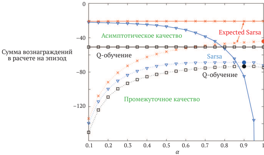
Рис. 6.3 ❖ Промежуточное и асимптотическое качество TD-методов управления в задаче о блуждании на краю обрыва в виде функции от \alpha . Во всех алгоритмах использовалась \varepsilon -жадная стратегия с \varepsilon = 0.1 . Асимптотическое качество получено усреднением по 100 000 эпизодов, а промежуточное – по первым 100 эпизодам. Эти данные получены усредненным по 50 000 и 10 прогонам для промежуточного и асимптотического случаев соответственно. Сплошными кружками обозначено наилучшее промежуточное качество каждого метода. Заимствовано из работы Seijen et al. (2009)
