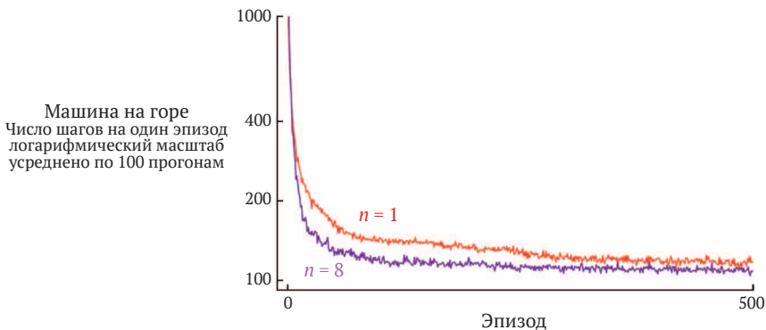
Рис. 10.3 ❖ Качество одношагового и 8-шагового полугradientного Sarsa в задаче о машине на горе. Использовались хорошие размеры шага: \alpha = 0.5/8 для n = 1 и \alpha = 0.3/8 для n = 8
