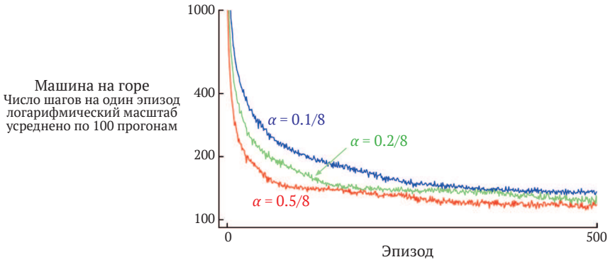
Рис. 10.2 ❖ Кривые обучения в задаче о машине на горе для полуградиентного метода Sarsa с аппроксимацией посредством плиточного кодирования и \epsilon -жадным выбором действий
