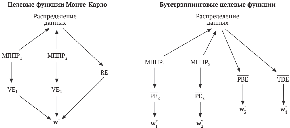
Рис. 11.4 ❖ Причинно-следственные связи между распределением данных, МППР и различными целевыми функциями. Слева – целевые функции Монте-Карло: два разных МППР могут порождать одно и то же распределение данных, но при этом иметь разные ошибки \overline{VE} , это доказывает, что целевую функцию \overline{VE} нельзя определить по данным, а стало быть, она необучаема. Однако у всех таких \overline{VE} должен быть один и тот же оптимальный вектор параметров w^* ! Более того, этот же вектор w^* можно найти с помощью другой целевой функции \overline{RE} , которая однозначно определяется по распределению данных. Таким образом, w^* и \overline{RE} обучаемы, хотя \overline{VE} – нет. Справа – бутстрэппинговые целевые функции: два разных МППР могут порождать одно и то же распределение данных и иметь разные минимизирующие векторы параметров; они необучаемы по распределению данных. Целевые функции \overline{PBE} и \overline{TDE} и их (различные) минимумы можно определить непосредственно по данным, т. е. они обучаемы
