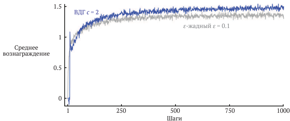
Рис. 2.4 ❖ Среднее вознаграждение за выбор ВДГ-действия на 10-руком испытательном стенде. Как видно, ВДГ, вообще говоря, работает лучше, чем \varepsilon -жадный выбор действия, за исключением первых k шагов, когда он случайно выбирает из еще не опробованных действий
