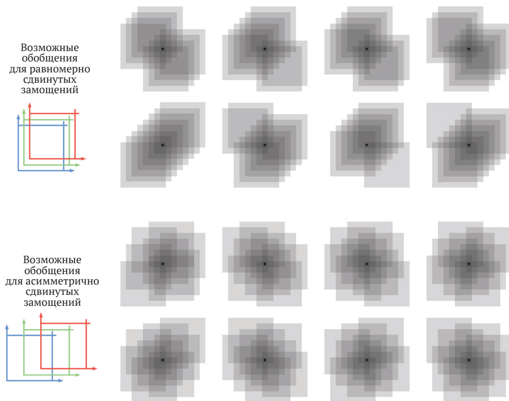
Рис. 9.11 ❖ Почему асимметричный сдвиг предпочтителен при плиточном кодировании. Показана сила обобщения обучающего состояния-примера, обозначенного черным знаком + , на близлежащие состояния для случая восьми замощений. Если замощения сдвинуты равномерно (сверху), то имеют место диагональные артефакты и заметные вариации обобщения, а если сдвиг асимметричный, то форма обобщения более однородна и похожа на сферу
