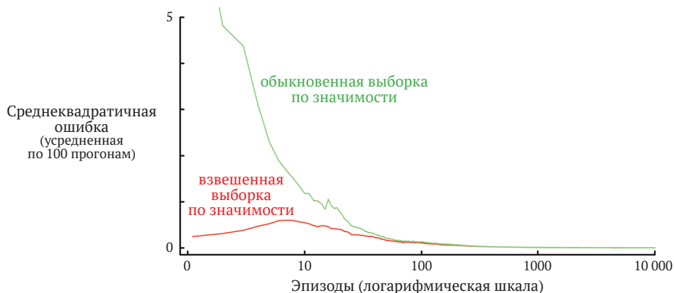
Рис. 5.3 ❖ Взвешенная выборка по значимости дает меньшую ошибку оценки ценности одного состояния в блэкджеке по эпизодам с разделенной стратегией ■
