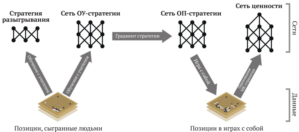
Рис. 16.6 ♠ Конвейер AlphaGo
