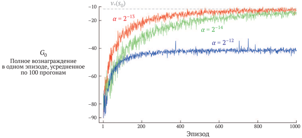
Рис. 13.1 ❖ Алгоритм REINFORCE для задачи о коротком коридоре в сеточном мире (пример 13.1). При удачно выбранном размере шага полное вознаграждение в одном эпизоде стремится к оптимальной ценности начального состояния
