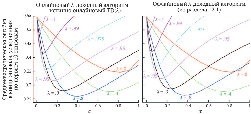
Рис. 12.8 ❖ Результаты для задачи о случайном блуждании с 19 состояниями (пример 7.1): показаны результаты онлайн- и офлайн- \lambda -доходных алгоритмов. В качестве меры качества здесь взята ошибка \sqrt{E} в конце эпизода, которая должна показывать наилучшие результаты для офлайн-алгоритма. Тем не менее онлайн-алгоритм работает немного лучше. Для сравнения, кривая, соответствующая \lambda = 0 , для обоих методов одинакова
