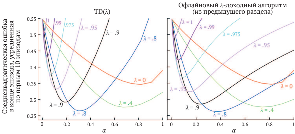
Рис. 12.6 ❖ Результаты для задачи о случайном блуждании с 19 состояниями (пример 7.1): показаны результаты TD( \lambda ) и офлайнного \lambda -доходного алгоритма. Оба алгоритма работают практически одинаково при небольших (меньших оптимального) значениях \alpha , но при больших \alpha TD( \lambda ) оказывается значительно хуже
