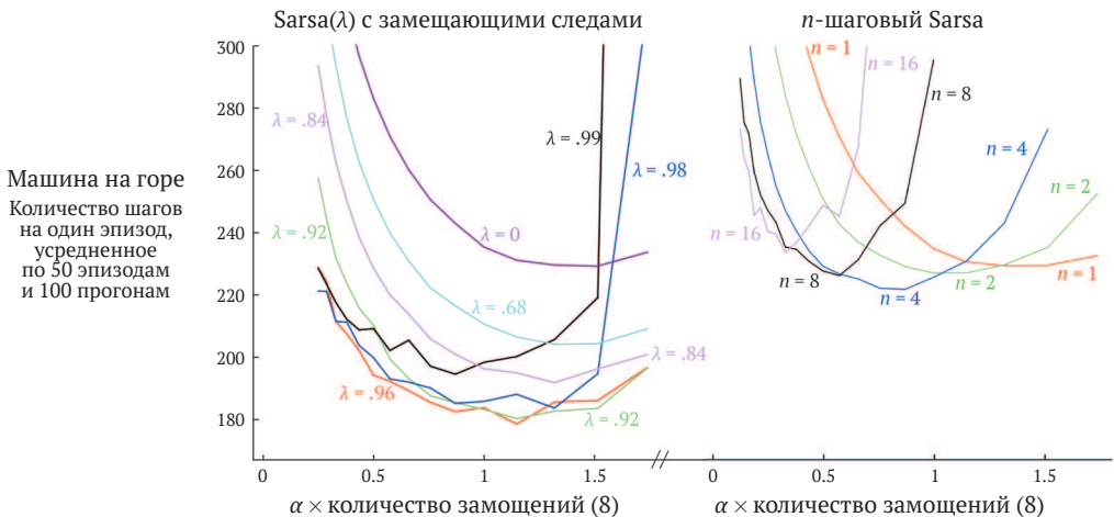
Рис. 12.10 ♦ Результаты работы двух алгоритмов для задачи о машине на горе – Sarsa( \lambda ) с замещающими следами и n -шагового Sarsa (повторение рис. 10.4) – в виде функции от размера шага
