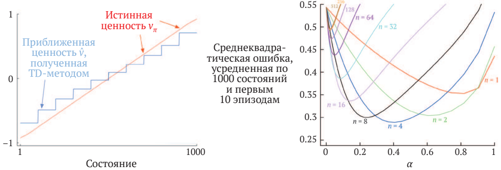
Рис. 9.2 ❖ Бутстрэппинг с агрегированием состояний в задаче о случайном блуждании с 1000 состояний. Слева: асимптотические ценности для полугradientного TD хуже, чем для метода Монте-Карло на рис. 9.1. Справа: результаты n -шаговых методов с агрегированием состояний поразительно напоминают полученные для табличного представления (см. рис. 7.2). Данные усреднены по 100 прогонам
