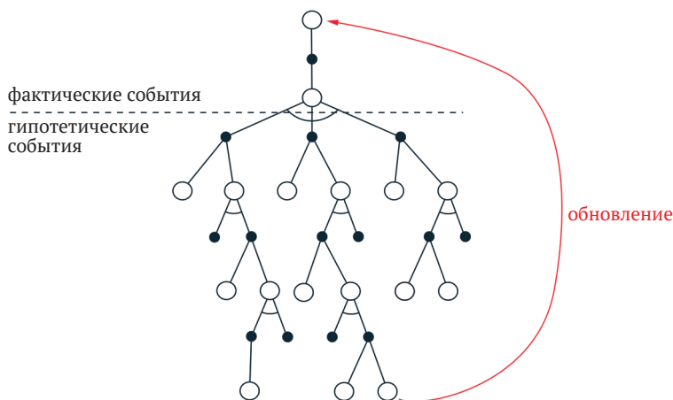
Рис. 16.2 ❖ Диаграмма предшествующих состояний для шашечной программы Сэмюэла
