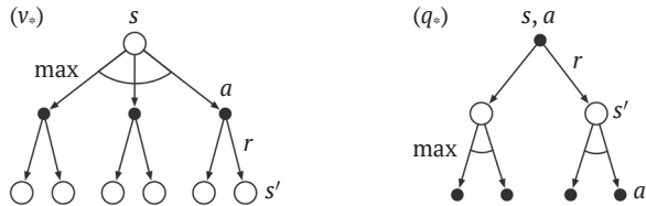
Рис. 3.4 ❖ Диаграммы предшествующих состояний для v_* и q_*
