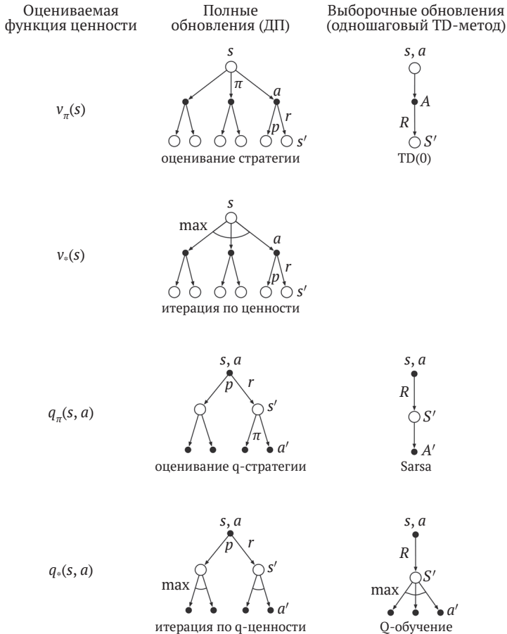
Рис. 8.6 ❖ Диаграммы предшествующих состояний для всех одношаговых обновлений, рассматриваемых в этой книге
