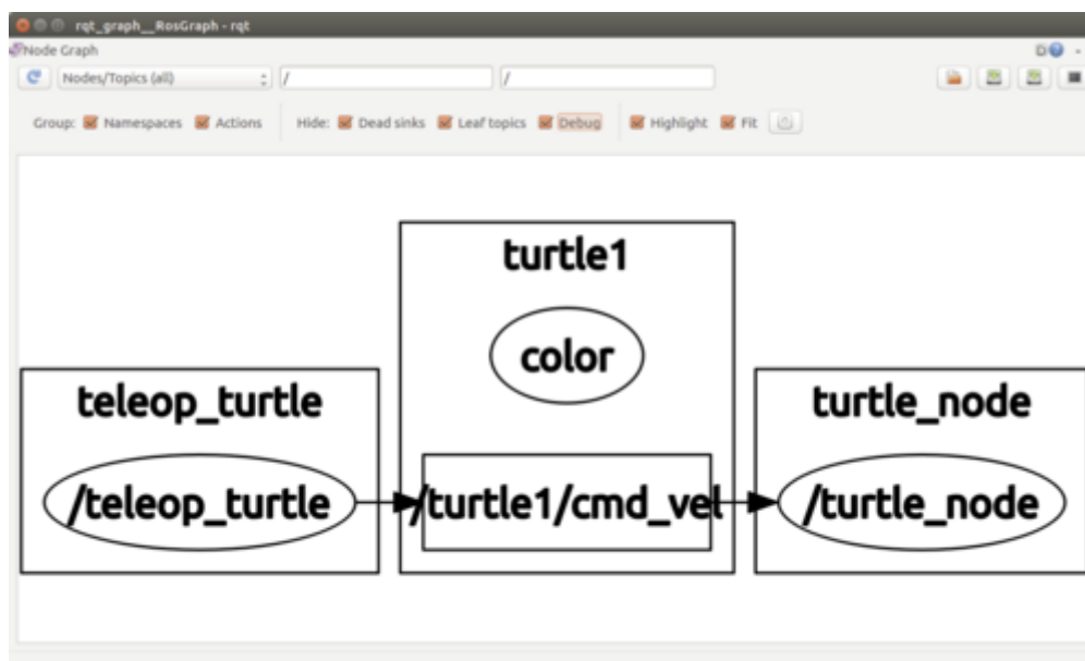
Рис. 3.4. Иллюстрация работы ноды типа rqt_graph.
