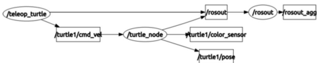
Рис. 3.3. Ноды /teleop_turtle , /turtle_node и /rosout и топики между ними.
