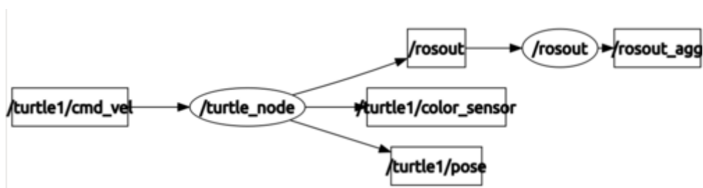
Рис. 3.2. Две ноды /turtle_node и /rosout и топики между ними.
